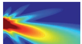
500Hz – DLA1244A+DLA804A
